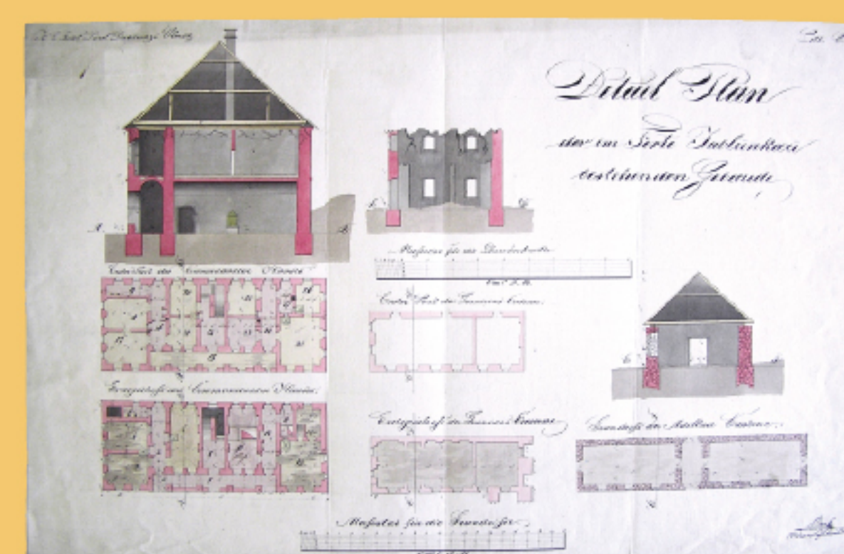
Podrobný plán budov stojacich v pevnosti Jablunkov vľavo: prvé poschodie a prizemie veliteľského domu vstrede: prvé poschodie a prizemie kasární pre posádku vpravo: pôdorys delostreleckých kasární
